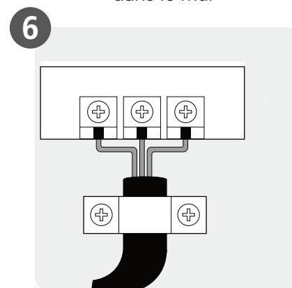
Connecter le câblage
