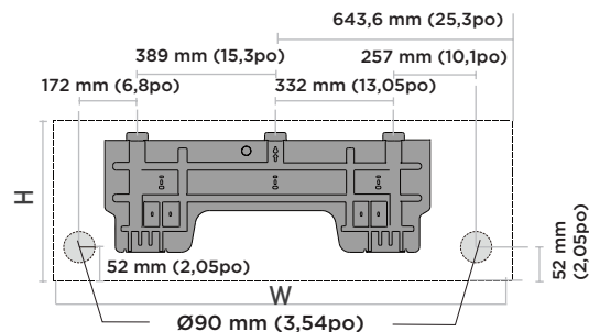
Dimensions de l'unité intérieure (L x H) : 1259 mm (49,55po) x 362 mm (14,25po)
