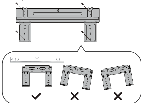
Orientation correcte de la plaque de montage
