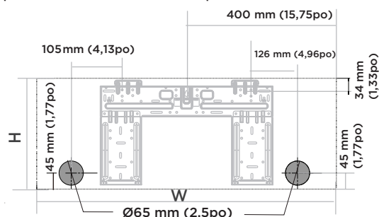
Dimensions de l'unité intérieure (L x H) : 729 mm (28,7po) x 293 mm (11,5po)
