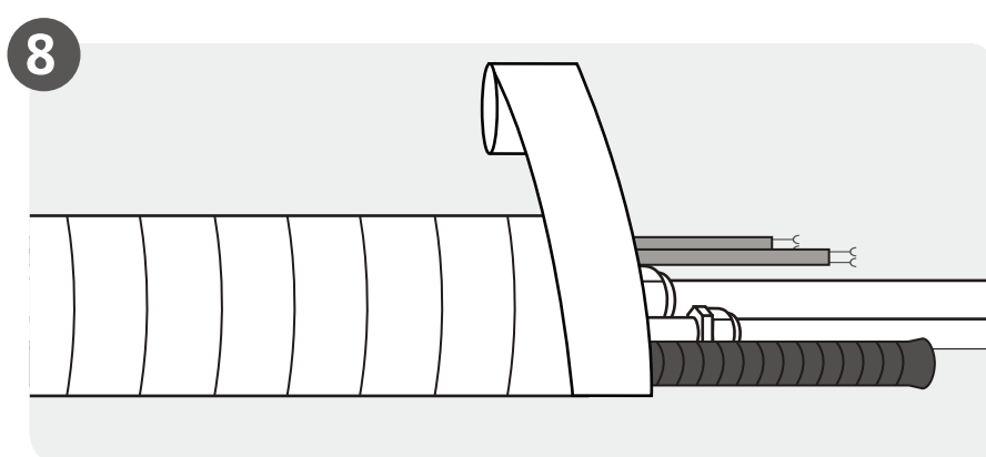
Envelopper les tuyaux et les câbles
