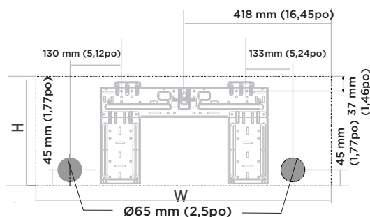
Dimensions de l'unité intérieure (L x H) : 835 mm (32,9po) x 296 mm (11,6po)
