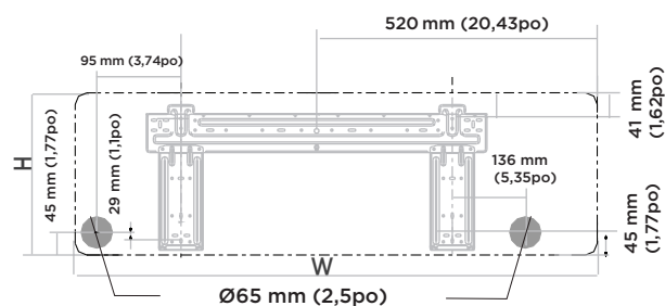
Dimensions de l'unité intérieure (L x H) : 971 mm (38,2po) x 321 mm (12,6po)
