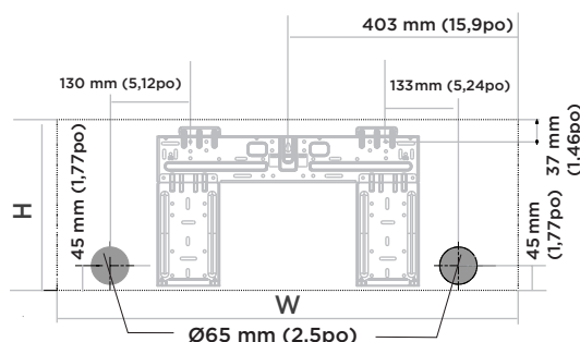
Dimensions de l'unité intérieure (L x H) : 806 mm (31,7po) x 296 mm (11,6po)
