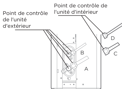
A : Vanne d'arrêt basse pression B : Vanne d'arrêt haute pression C ET D : Écrous évasés de l'unité d'intérieur
