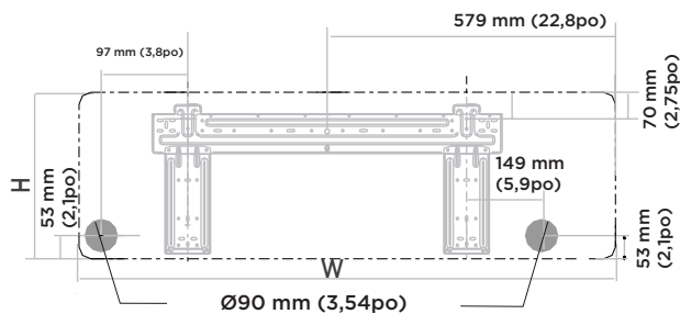
Dimensions de l'unité intérieure (L x H) : 1082 mm (42,6po) x 338 mm (13,3po)
