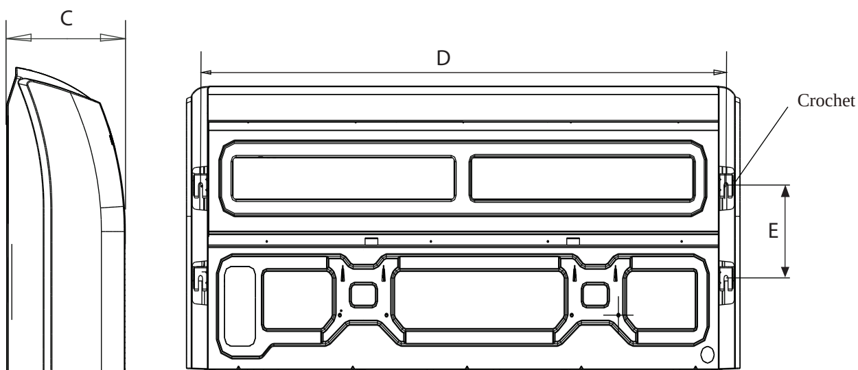
Taille de l'installation des pièces intérieures
