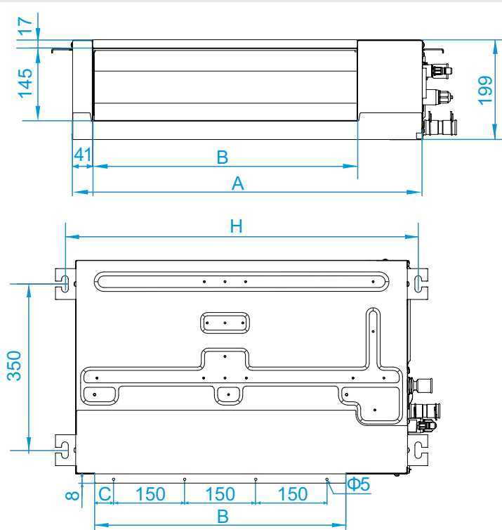
Taille de l'entrée d'air de retour (mode d'air de retour arrière) :
