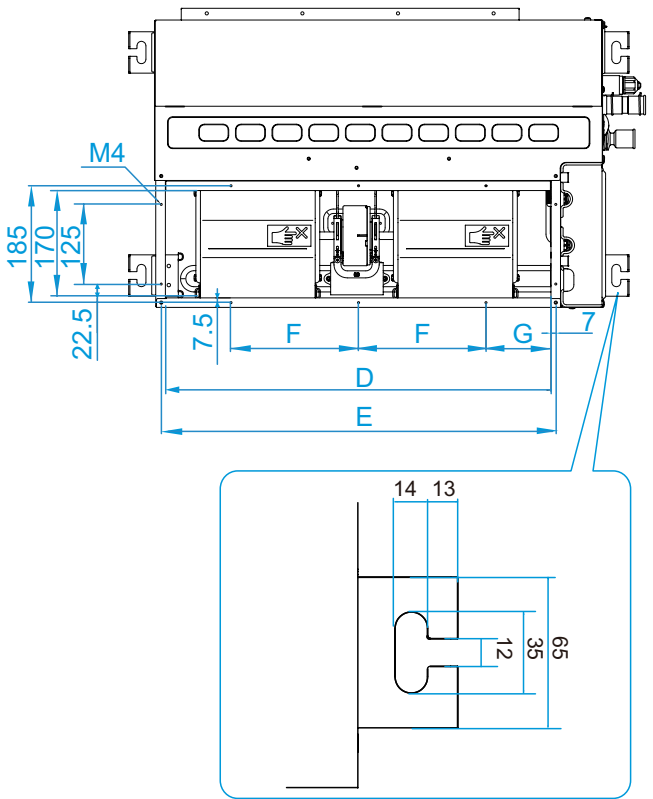
Taille de l'entrée d'air de retour (mode de retour d'air par le bas) et distance entre les cosses :
