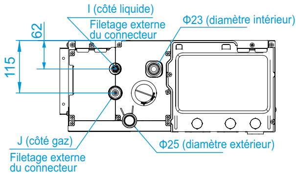
Dimension du tuyau et de la conduite d'eau :
