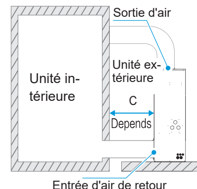
Sortie supérieure-Retour d'air arrière
