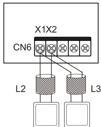
Deux contrôleurs pour une unité intérieure (le contrôleur câblé maître-esclave doit être configuré. Pour plus de détails, voir le manuel du contrôleur câblé)
