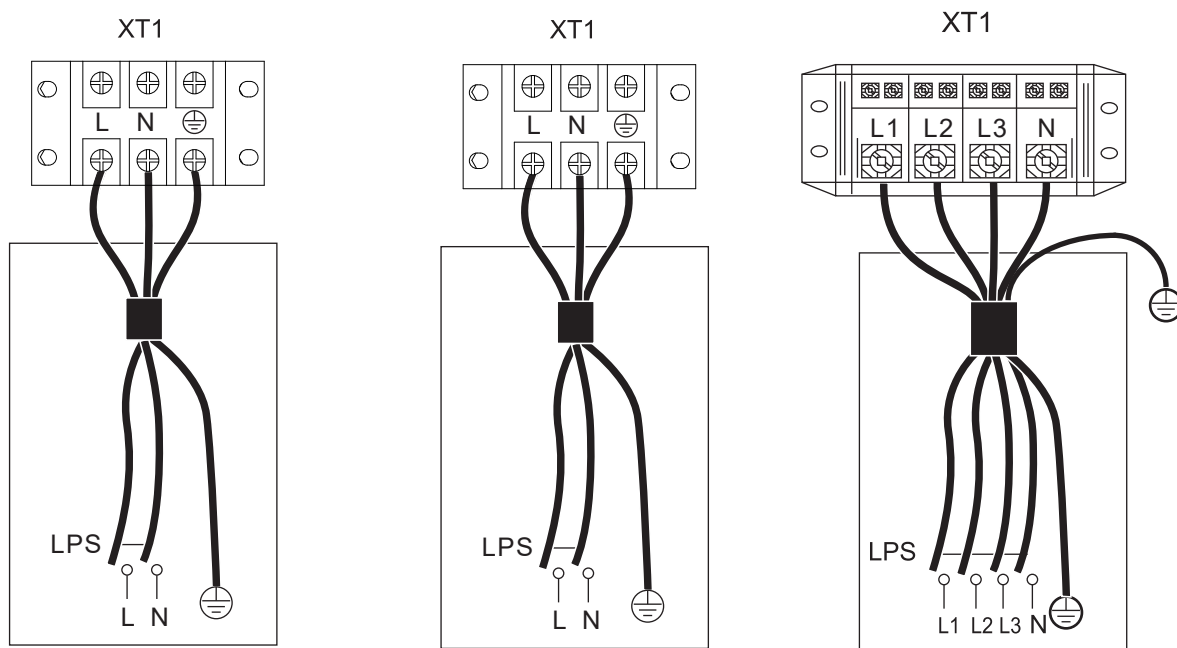
ALIMENTATION DE L'UNITÉ INTÉRIEURE Réchauffeur de secours de 3 kW monophasé standard
